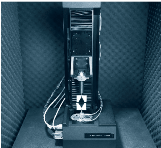
T150 UTM
